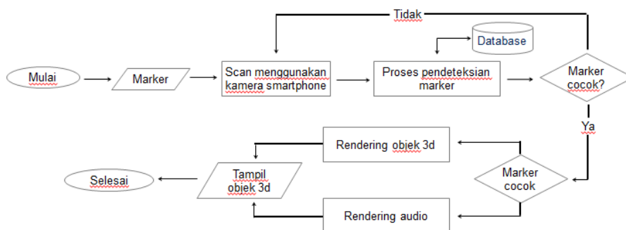
Gambar 2. Flowchart aplikasi
