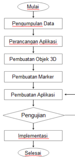
Gambar 1. Metode perancangan
