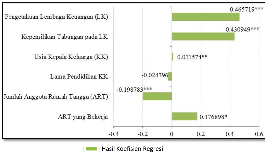
Keterangan: ***: \alpha 0.01; **: \alpha 0.05; *: \alpha 0.10 Gambar 1. Grafik Analisis Regresi Linier dengan Variabel Dummy Sumber: Data primer diolah, 2021
