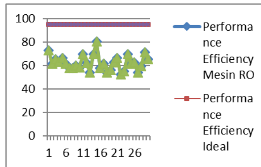
Gambar 4.7 Grafik Performance Efficiency Pada Mesin RO Mulai Tanggal 1 Sampai 30 November 2017
