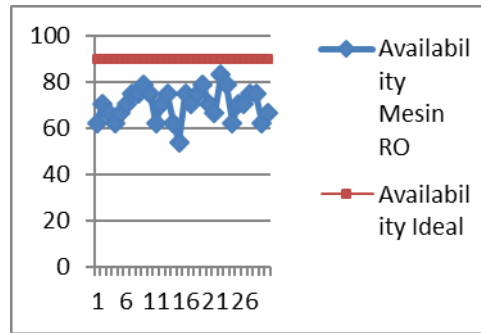
Gambar 4.6 Grafik Hasil Perhitungan Availability Pada Mesin RO mulai tanggal 1 sampai 30 november
