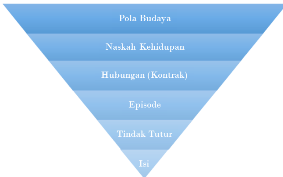
Gambar 2. Hierarki CMM
